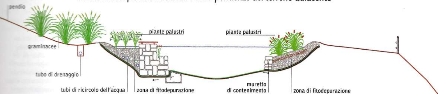
Sezione della piscina naturale e delle pendenze del terreno adiacente
